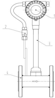
图 1 KSDLU-GB 液氧、液氮、液氩专用流量计产品结构
